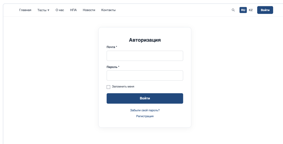
Рисунок 2 — Авторизация
