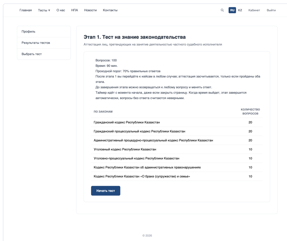
Рисунок 7 — Правила этапа 1
