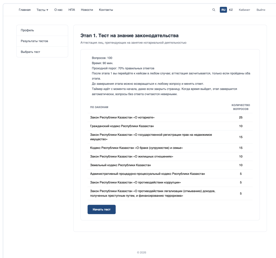
Рисунок 7 — Правила этапа 1
