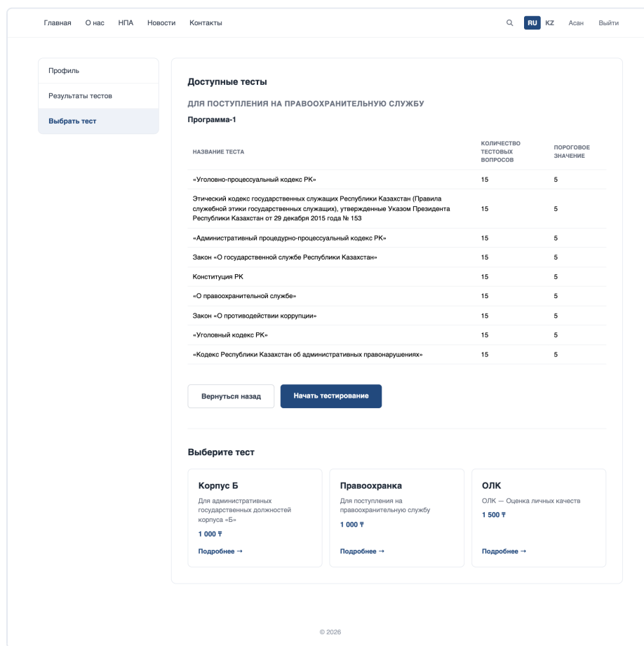
Рисунок 8 — Начало тестирования
