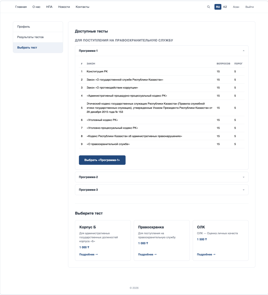
Рисунок 7 — Выбор программы
