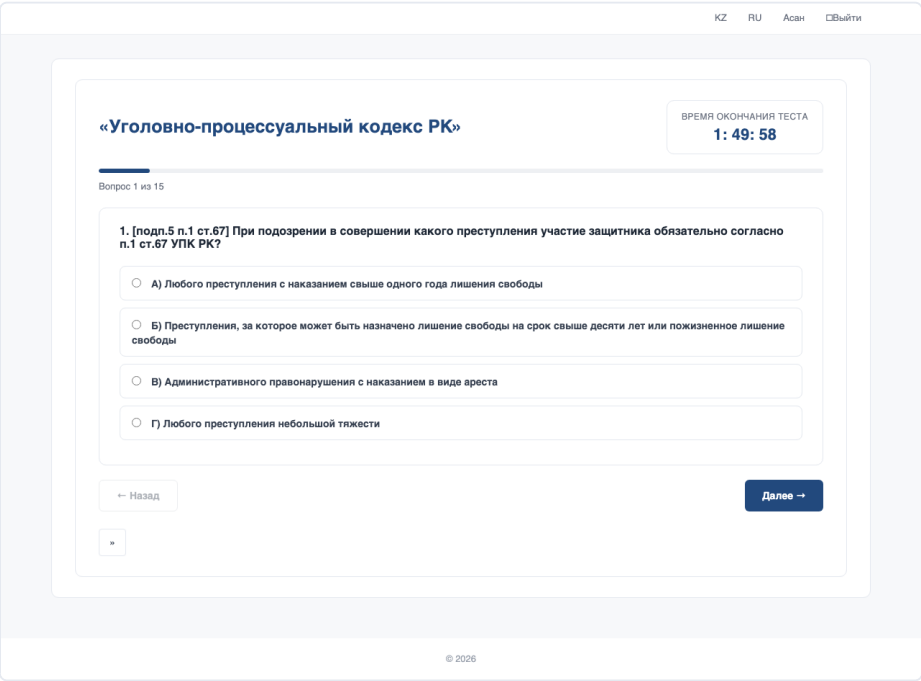
Рисунок 9 — Прохождение теста
