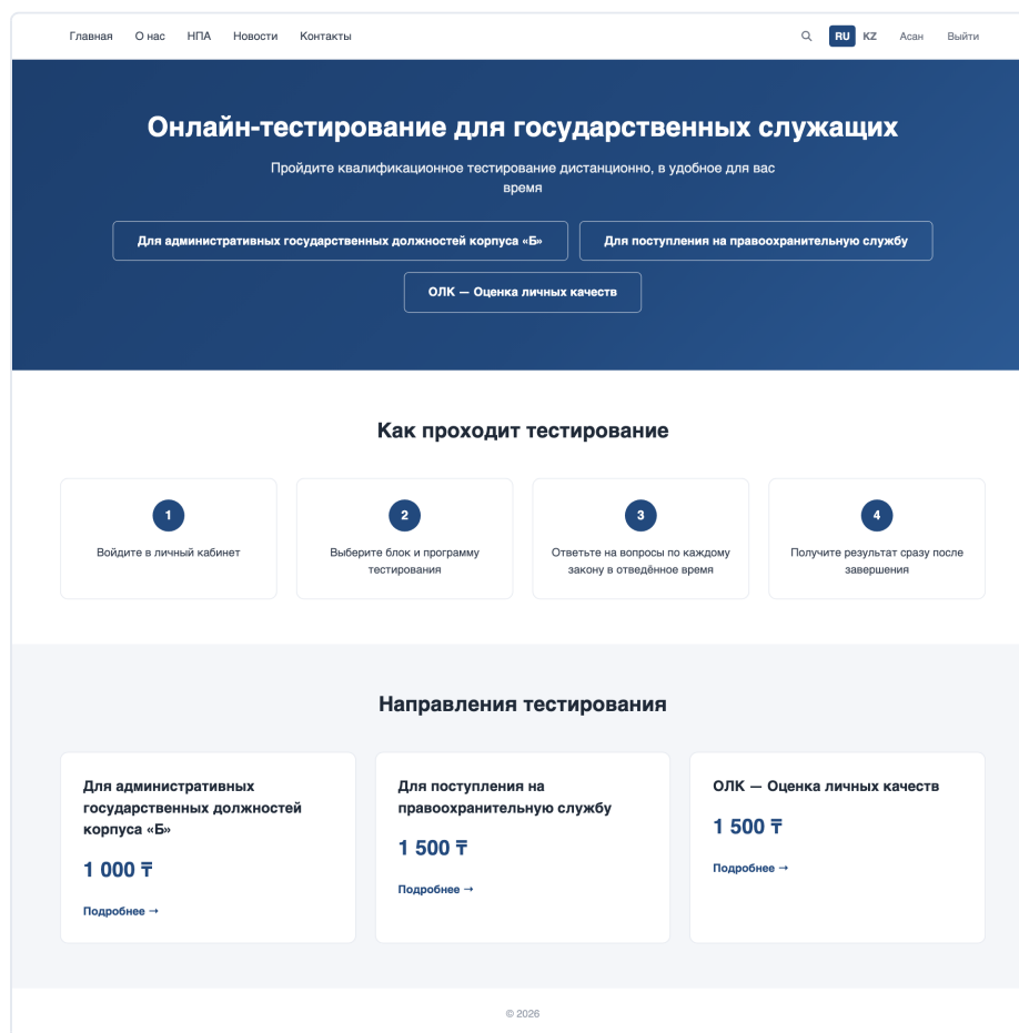
Рисунок 3 — Главная страница
