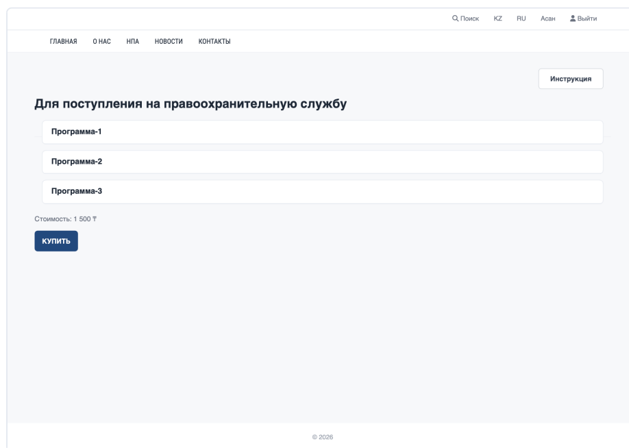
Рисунок 4 — Страница теста
