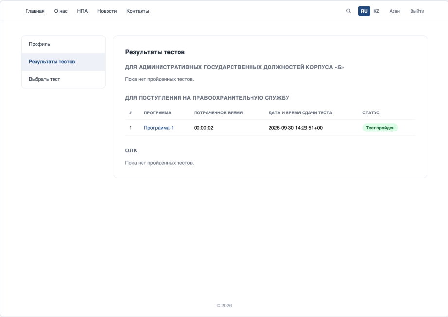
Рисунок 10 — Результаты тестов
